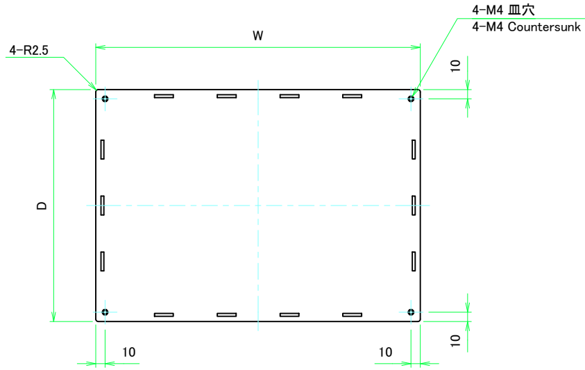
上カバー表面 / Top cover Frontside
