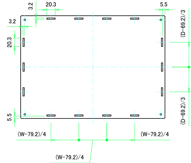
上カバー裏面 / Top cover Backside
