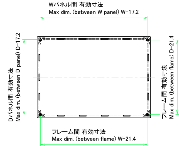
下カバー / Bottom cover
